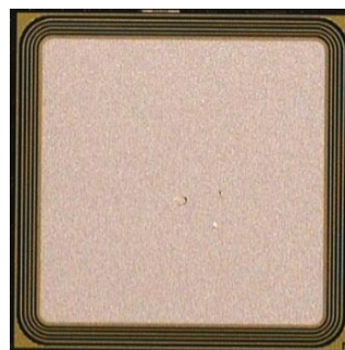
芯片示意图 Die View
